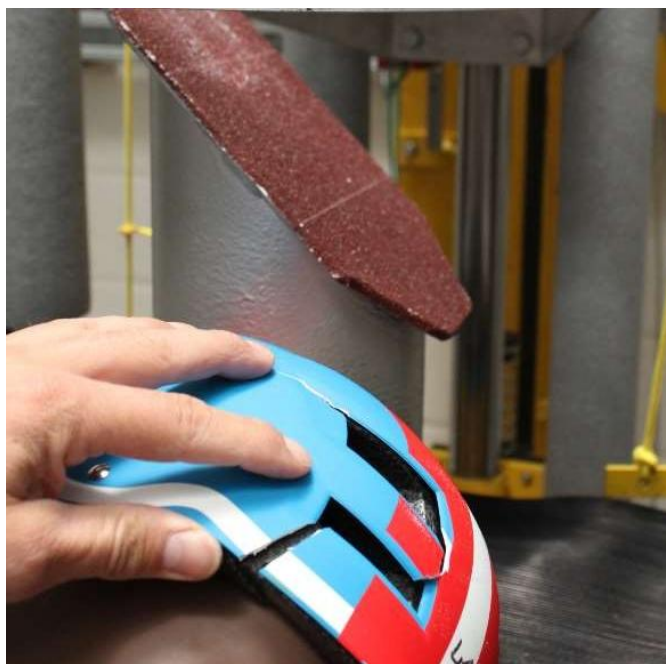
Slika 1: ABS vanjska školjka napukne u gotovo svim testovima apsorpcije udara
