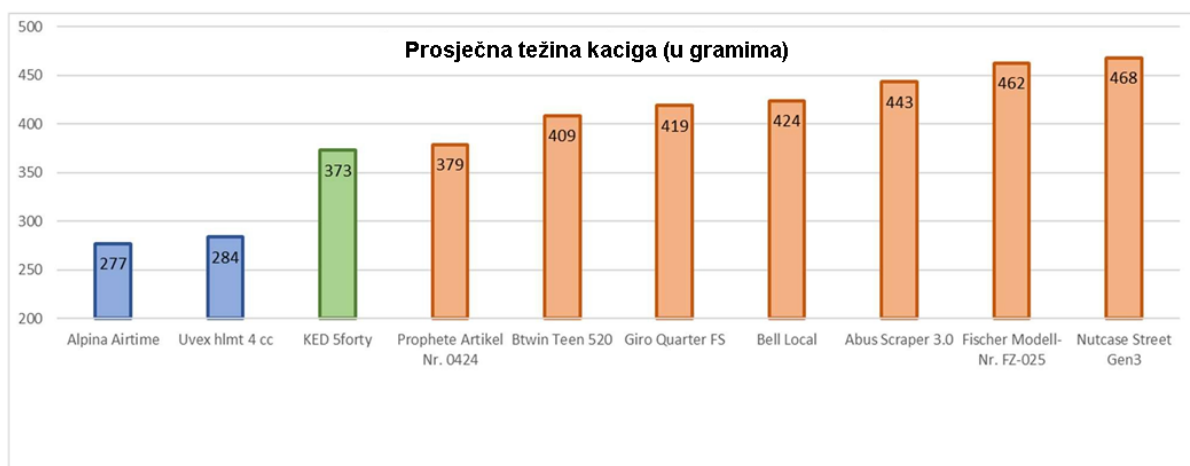
Slika 5: Težina testiranih biciklističkih kaciga; boja označava tehnologiju konstrukcije
