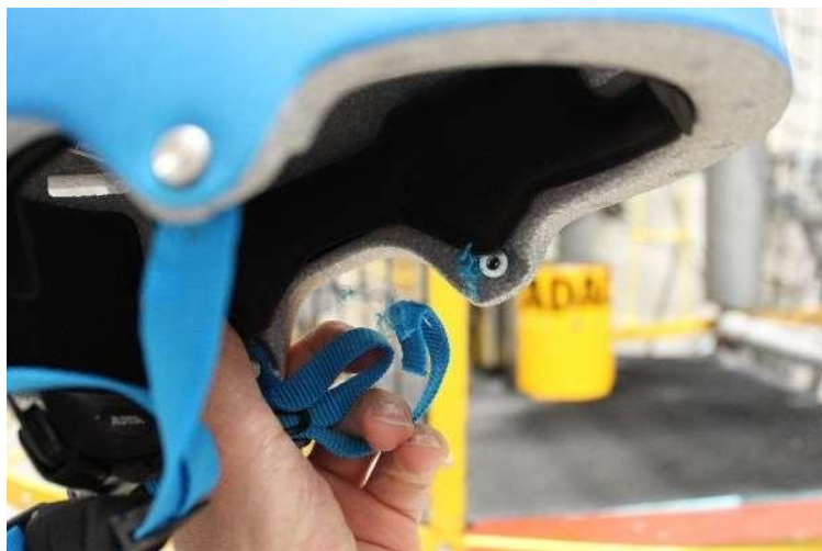
Slika 2: Veza za remen udovoljava standardnim zahtjevima, ali ne podnosi dodatna opterećenja
